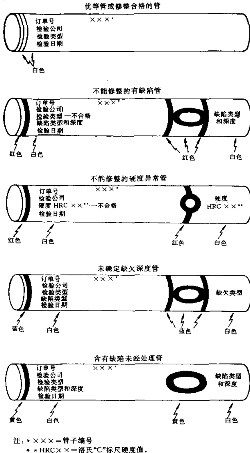
图 2 新管线管的检验标志
