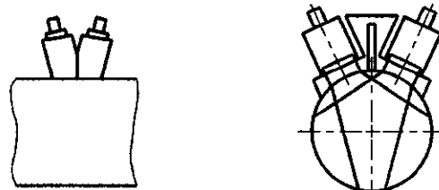
双晶纵波探头
