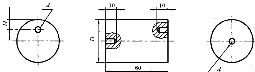
图 4 短横孔标准人工缺陷试块加工图
