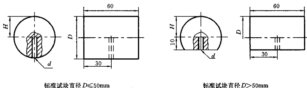
图 5 平底孔标准人工缺陷试块加工图
